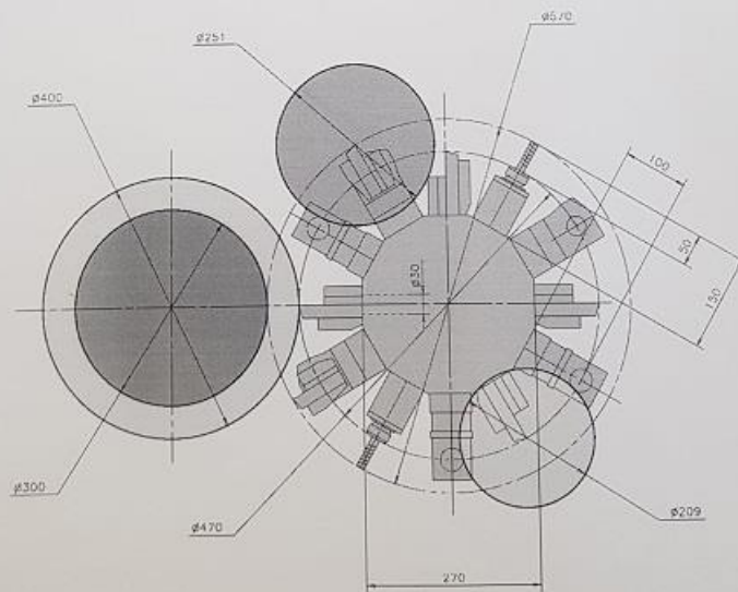
Abbildung 3-8: Arbeitsraumabmessungen
